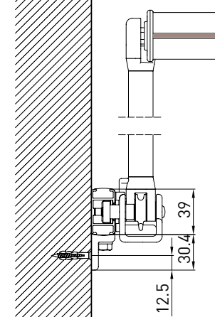
guida a nicchia - niche guide B-B
