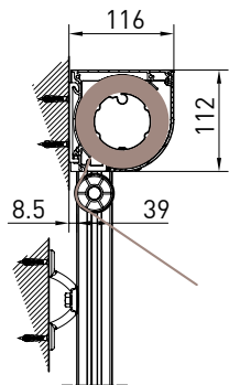
TONDO - ROUND A-A
