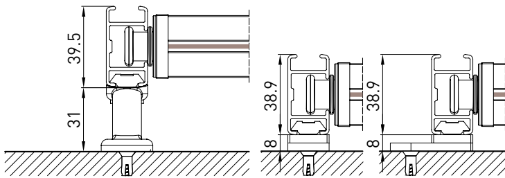
guida a parete - wall guide B-B
