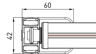
guida a pavimento - floor guide B-B
