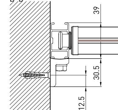
guida a nicchia - niche guide B-B
