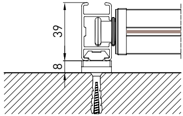
guida a parete - wall guide B-B
