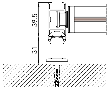
guida a parete - wall guide B-B
