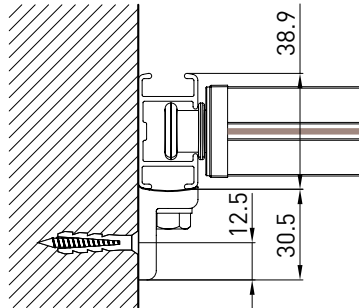
guida a nicchia - niche guide B-B
