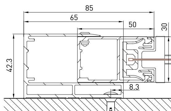
Guida a parete (GCP) - Wall guide (GCP) Coulisse façade (GCP) - Wandführung (GCP) B-B
