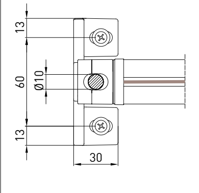
piedino a pavimento - floor bracket B-B
