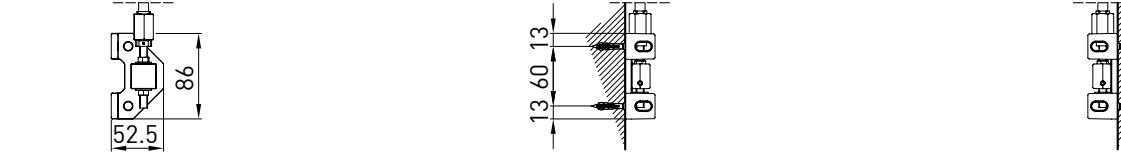
Piedino a pavimento - Floor foot - Pied sol - Bodenbefestigung
