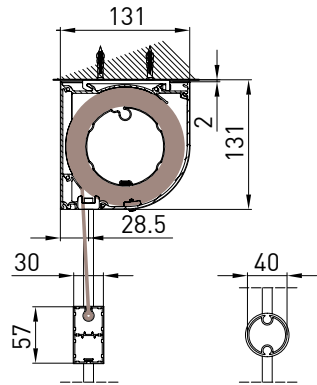
TONDO - ROUND A-A
