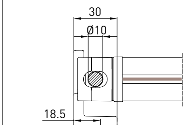
supporto a nicchia - niche bracket B-B
