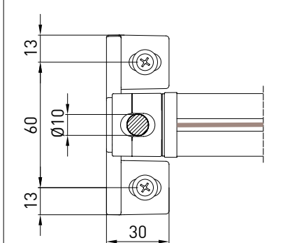
piedino a pavimento - floor bracket B-B
