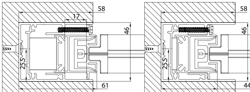
Guida a nicchia - Niche guide Coulisse tableau - Nischenführung B-B
