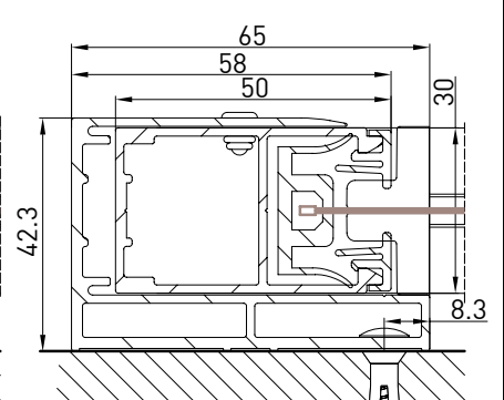
Guida a parete (GCP) - Wall guide (GCP) Coulisse façade (GCP) - Wandführung (GCP) B-B
