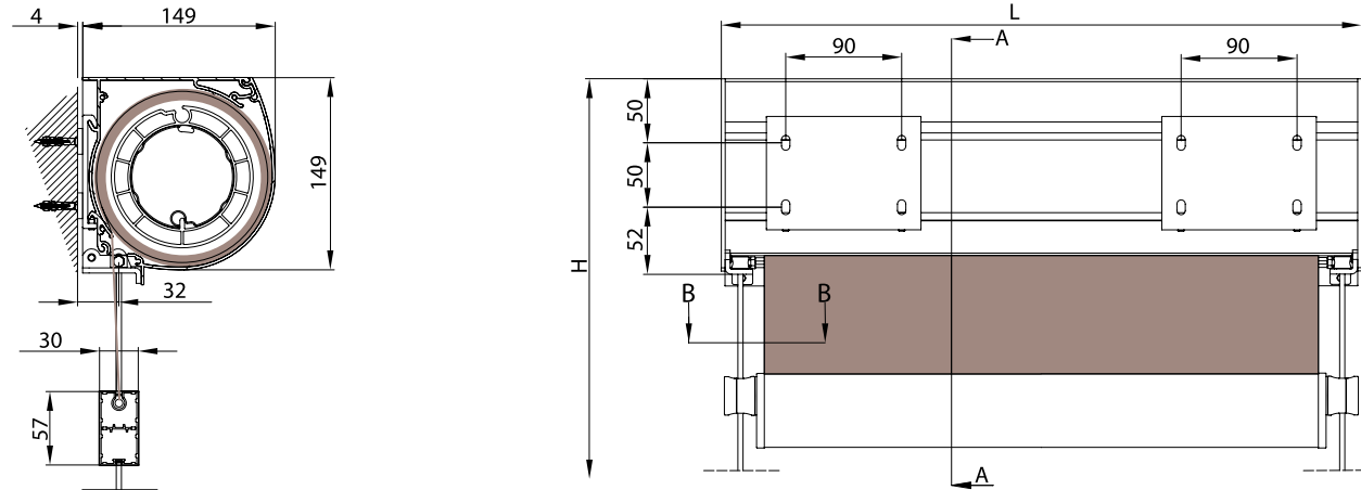
supporto a parete - wall bracket
