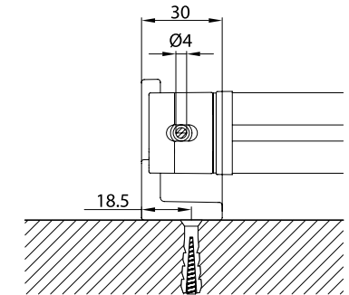
supporto a nicchia - niche bracket B-B
