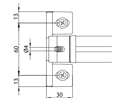
pedino a pavimento - floor bracket B-B
