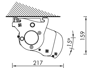
Installazione a soffitto 15° Ceiling installation 15°
