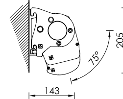
Installazione a parete 75° Wall installation 75°
