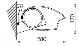
Installazione a parete Wall installation
