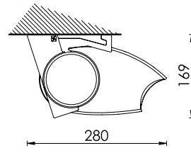
Installazione a soffitto Ceiling installation
