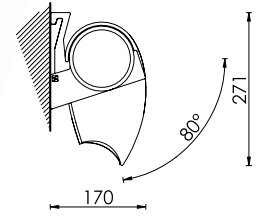
Installazione a parete 80° Wall installation 80°
