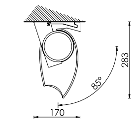
Installazione a soffitto 85° Ceiling installation 85°
