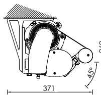
Installazione a soffitto 45° Ceiling installation 45°
