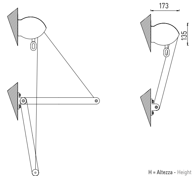
Installazione a parete con tettuccio Wall installation with a hood
