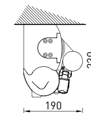
Installazione a soffitto Ceiling installation
