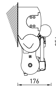
Installazione con bracci incrociati Crossed arms installation
